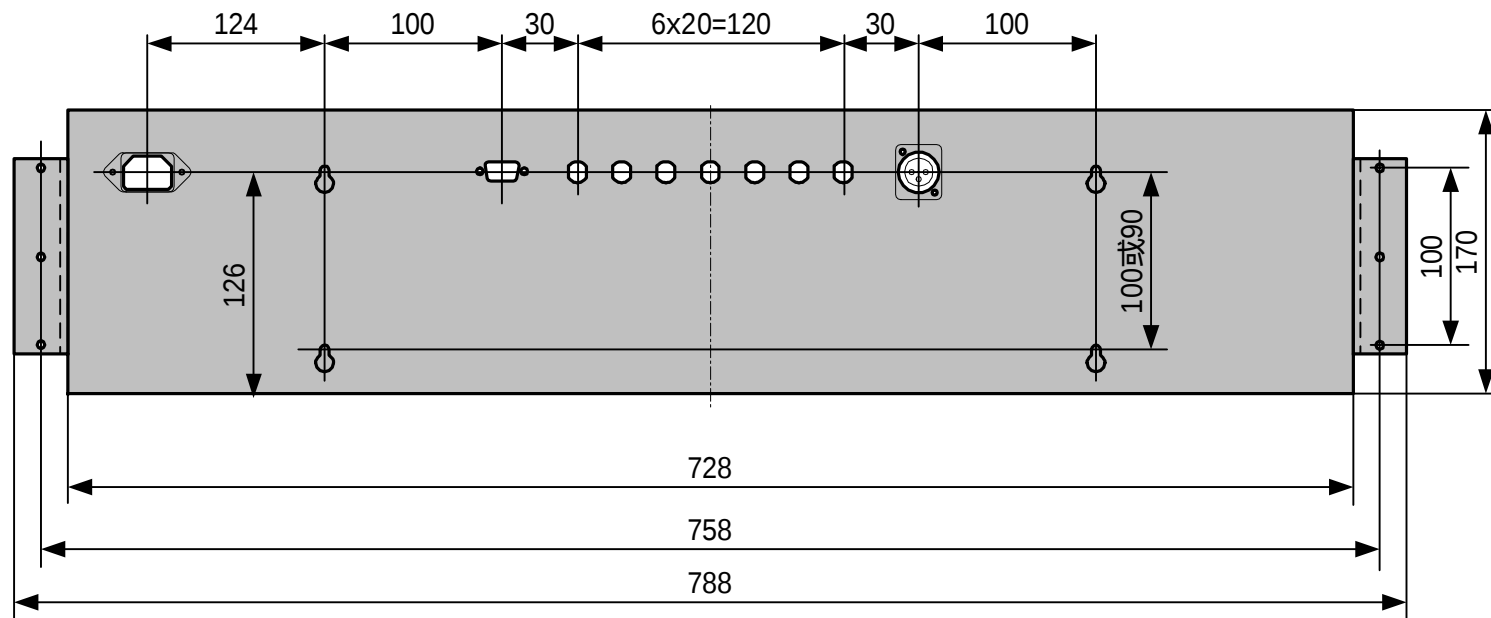
电视墙开孔示意图
